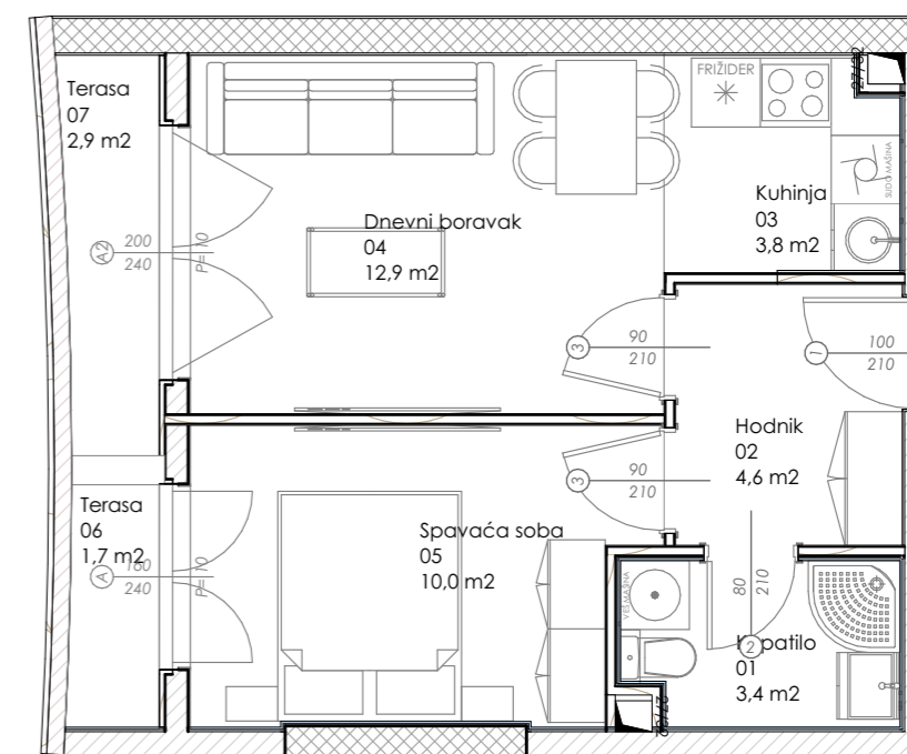
ORGANIZACIJA STANA L1-X-J3
